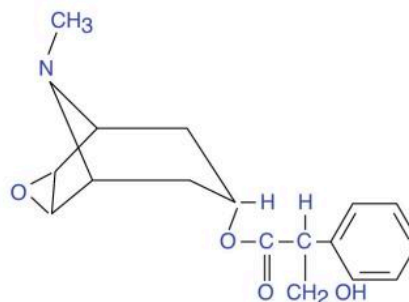
Scopolamine (Hyoscine)
