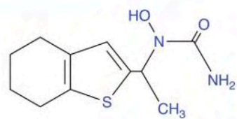
Zileuton
