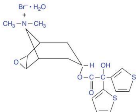
Tiotropium bromide
